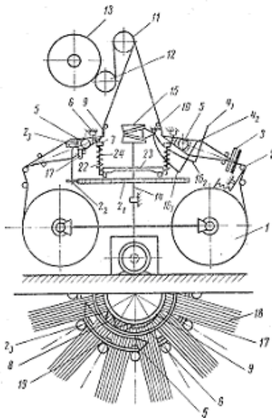
Расми 97. Нақшаи дастгоҳи мудаавари ТКД-425-Л.
