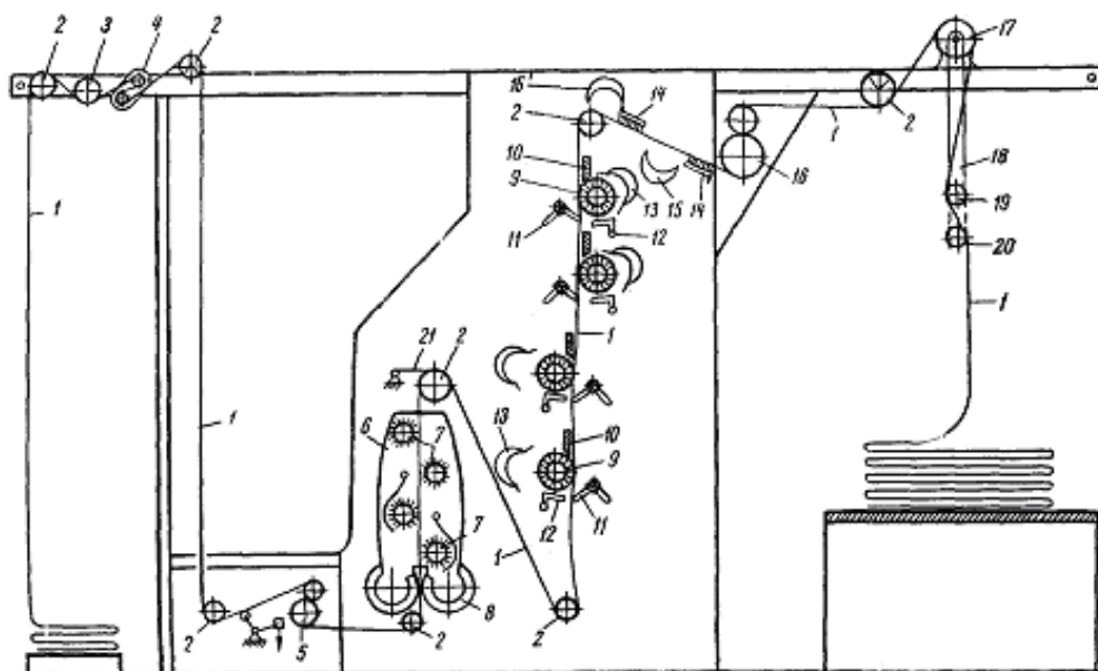
Расми 114. Нақшаи технологии мошини тозакунандаю тарошанда УСД
