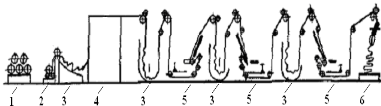
Расми 115. Нақшаи ҷойгиршавии таҷҳизот дар хати муттасили агрегатӣ
