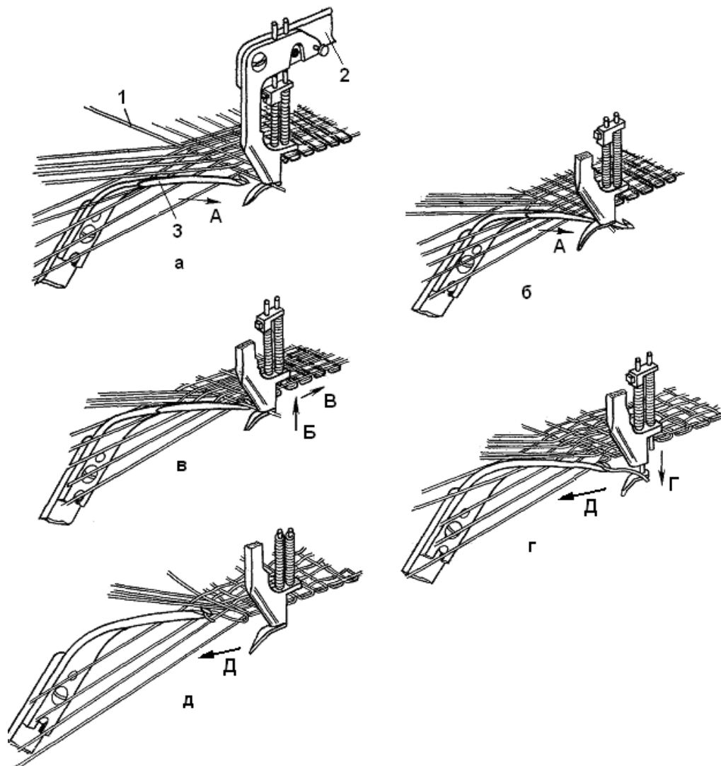
Расми 107. Тартиби ҳошиябандӣ бо усули каткунӣ
