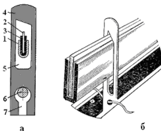
Расми 109. Нақшаи назораткунандаи ресмонҳои тори дастгоҳи дорои пудгузаронакҳо
