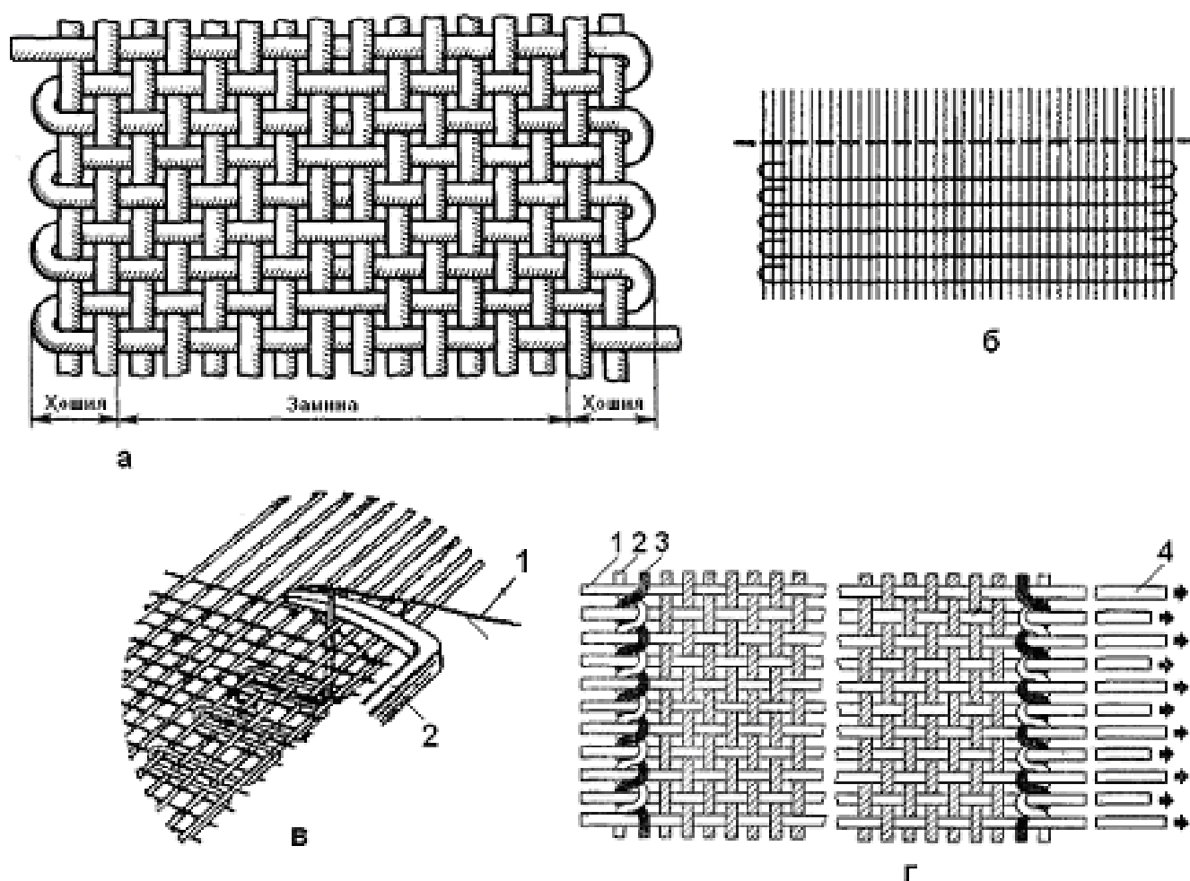
Расми 106. Тарзҳои гуногуни ҳошиябандӣ
